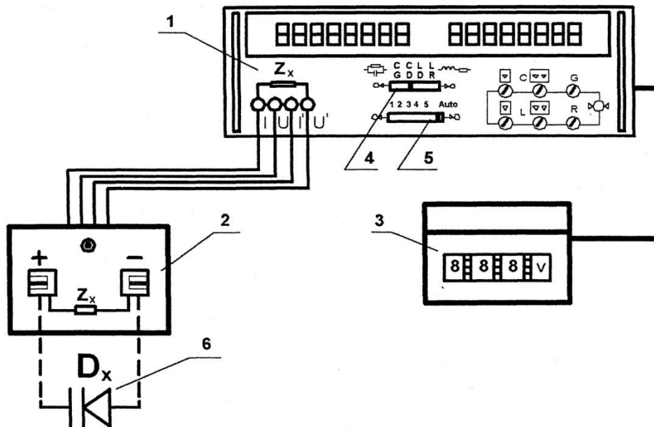
Rys. 1. Schemat stanowiska do przeprowadzania pomiarów charakterystyk napięciowo - pojemnościowych warikapów
